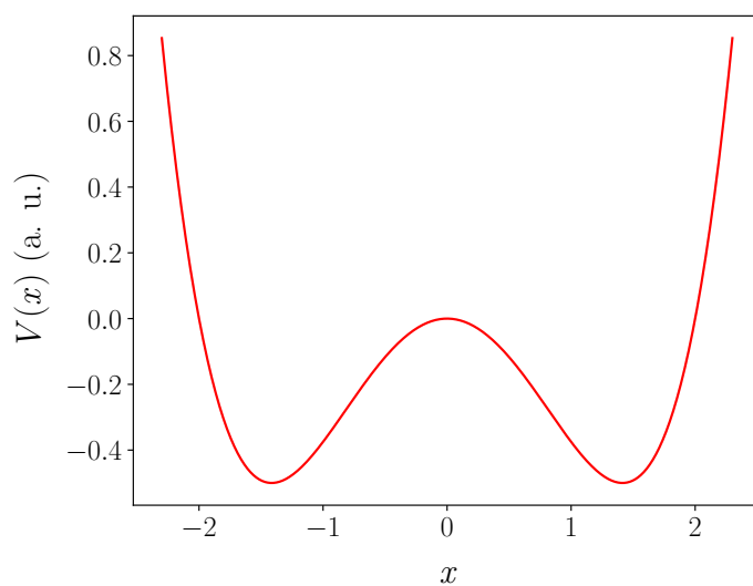
Graf 3: Klasický potenciál V(x) (??) s parametry a = b = 1
